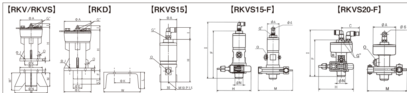
■ Dimensions (mm)
