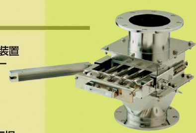
テツキャッチャー
